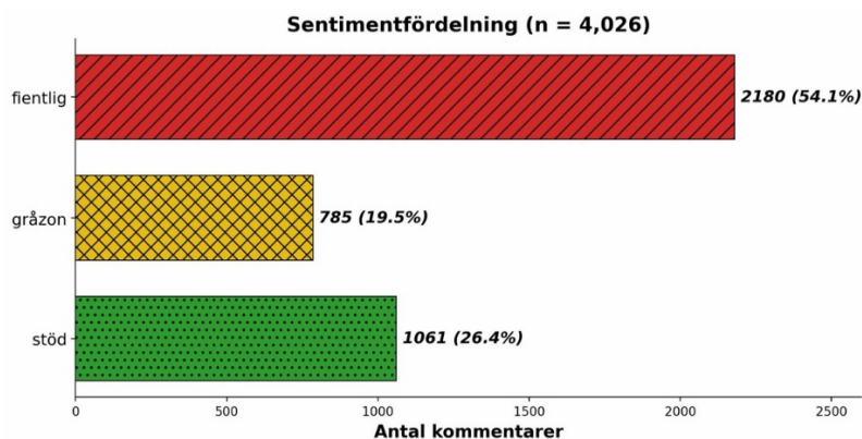
Figur 2. Sentimentfördelning
