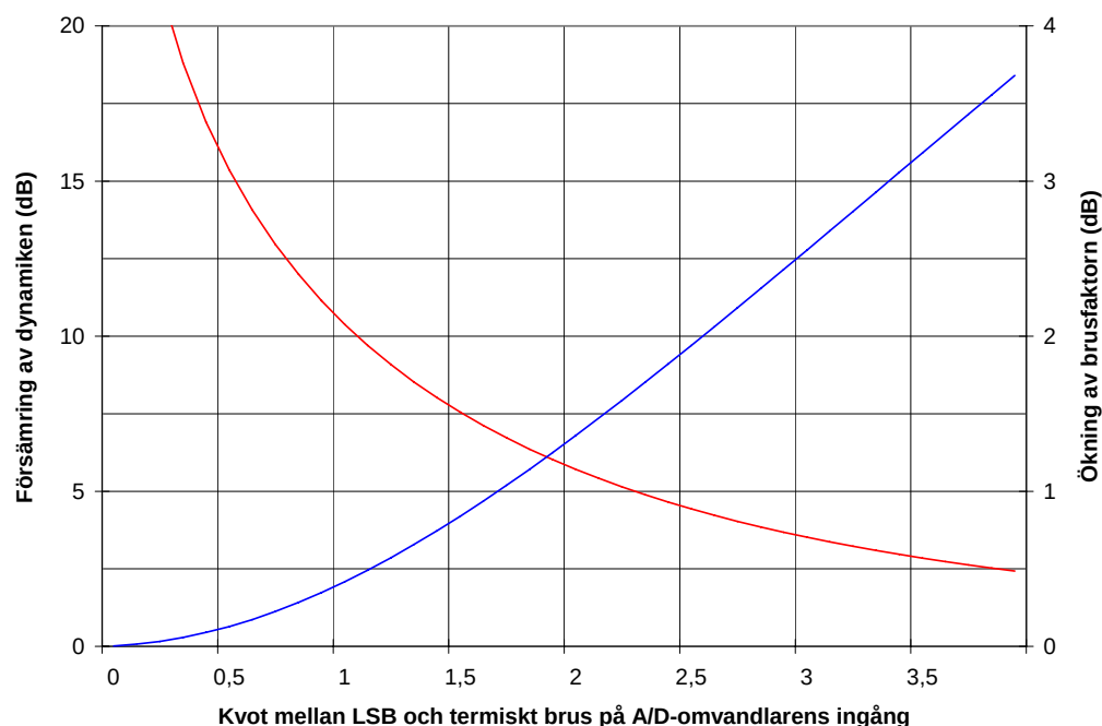
Figur 16 Storleken på förstärkningen i mottagarens analoga frontend är en kompromiss som påverkar mottagarens dynamik respektive känslighet. Med låg förstärkning är kvoten mellan en LSB i digitaliseringen och inbrusnivån till A/D-omvandlaren stor, vilket leder till bra dynamik men dålig känslighet. I diagrammet framgår detta genom en ökning av brusfaktorn.
