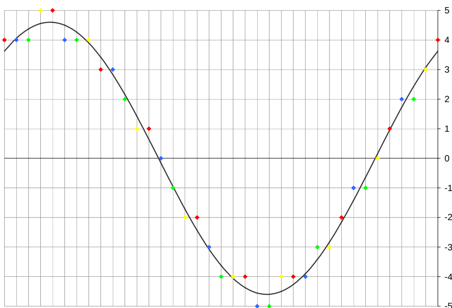
Figur 11 Principen för tidsinterleaving av A/D-omvandlare är enkel. I det visade fallet samplar fyra likadana omvandlare insignalen med samma samplingsfrekvens. Samplingstidpunkterna är dock förskjutna så att hela samplingsmängden tillsammans motsvarar vad som fås med en A/D-omvandlare och fyra gånger högre samplingsfrekvens. I figuren visas sampel från respektive A/D-omvandlare med olika färg.
