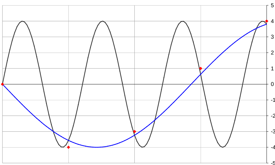
Figur 6 Om den högre frekvensen höjs något, relativt i figur 5, finns det fortfarande en lägre frekvens som ger exakt samma sampelsekvens. Till skillnad mot i föregående exempel ger vissa samplingstidpunkter här ett kvantiseringsfel.
